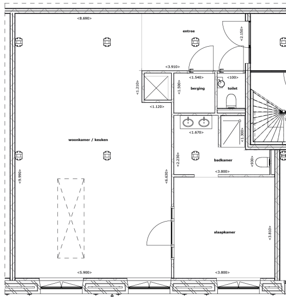
Plattegrond verdieping 01 1:50
